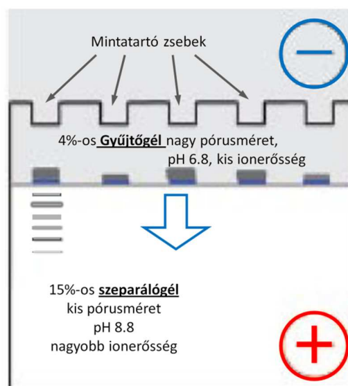
7. ábra Az SDS-PAGE gél felépítése
