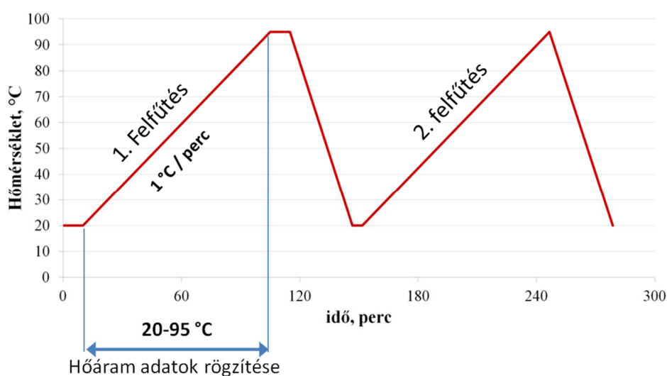
20. ábra Az alkalmazott DSC hőmérséklet-program grafikus képe
